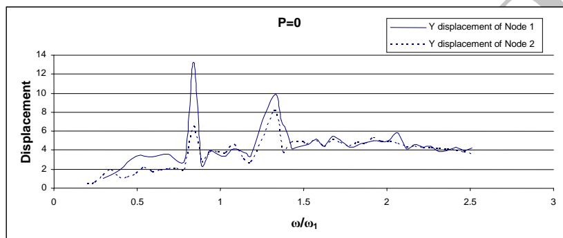
شکل ۲۳- بزرگنمایی مؤلفه Y میدان جابه‌جایی سطحی سربز نیلوفری با در نظر گرفتن اندرکنش آن با پی در دو گره ۱ و ۲ تحت برخورد موج P با زاویه و آزیموت صفر درجه
