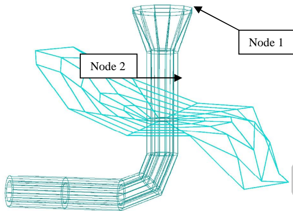
شکل ۱۸- نمایشی از سرریز نیلوفری و پی اطراف آن
