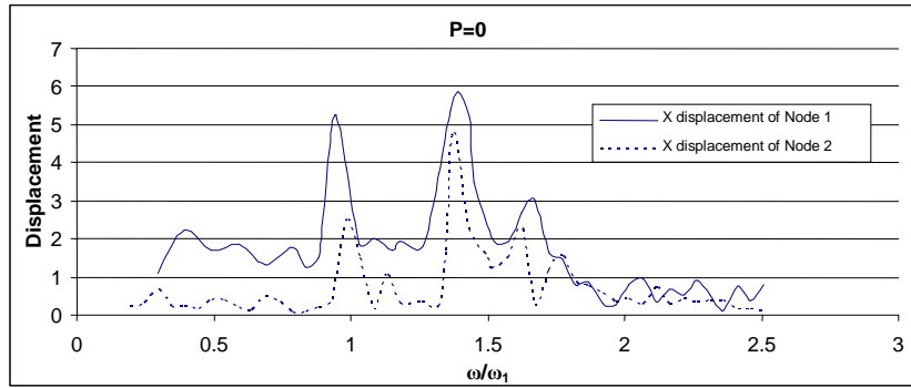
شکل ۲۲- بزرگنمایی مؤلفه X میدان جابه‌جایی سطحی سربز نیلوفری با در نظر گرفتن اندرکنش آن با پی در دو گره ۱ و ۲ تحت برخورد موج P با زاویه و آزیموت صفر درجه
