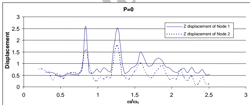
شکل ۲۴- بزرگنمایی مؤلفه Z میدان جابه‌جایی سطحی سربز نیلوفری با در نظر گرفتن اندرکنش آن با پی در دو گره ۱ و ۲ تحت برخورد موج P با زاویه و آزیموت صفر درجه
