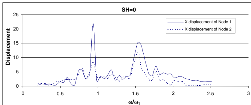
شکل ۲۵- بزرگنمایی مؤلفه X میدان جابه‌جایی سطحی سربز نیلوفری با در نظر گرفتن اندرکنش آن با پی در دو گره ۱ و ۲ تحت برخورد موج SH با زاویه و آزیموت صفر درجه
