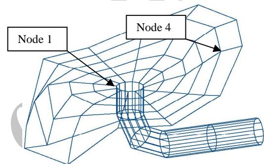
شکل ۱۴- هندسه و نحوه المان‌بندی خاک اطراف سرریز
