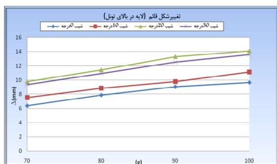
شکل ۱۳- نمودار تغییر شکل قائم در شیب‌های مختلف برای میان لایه در بالای تونل
