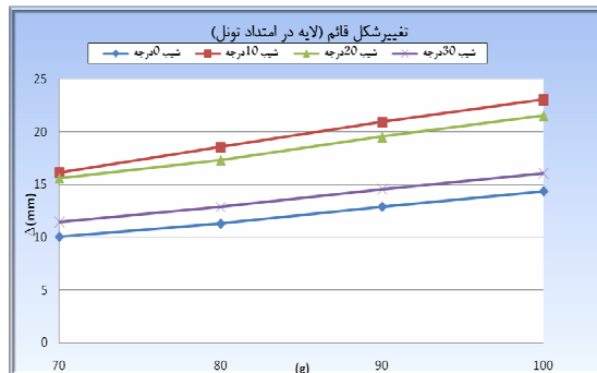
شکل ۱۱- نمودار تغییر شکل قائم در شیب‌های مختلف برای میان لایه در امتداد تونل
