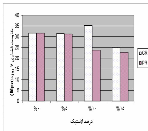
شکل ۴- مقایسه مقاومت فشاری ۷ روزه بتن‌های حاوی خرده لاستیک و پودر لاستیک
