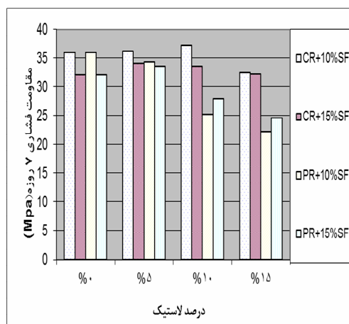
شکل ۶- مقایسه مقاومت فشاری ۷ روزه بتن‌های حاوی خرده لاستیک و پودر لاستیک به همراه ۱۰ و ۱۵ درصد میکروسیلیس
