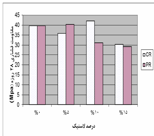
شکل ۵- مقایسه مقاومت فشاری ۲۸ روزه بتن‌های حاوی خرده لاستیک و پودر لاستیک
