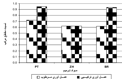
شکل ۲۵- نسبت مقطع مرکب تیرهای خمشی با سطح تماس زبر
