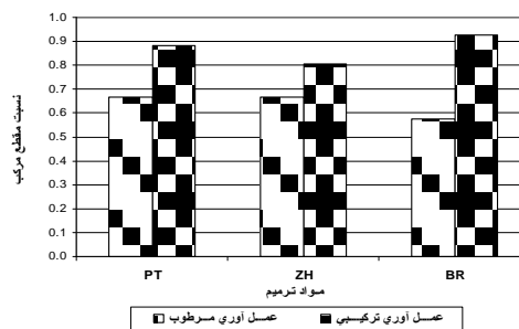
شکل ۲۴- نسبت مقطع مرکب تیرهای خمشی با سطح تماس صاف
