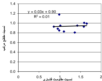
شکل ۲۱- رابطه نسبت مقاومت فشاری با نسبت مقطع مرکب در شرایط عمل آوری ترکیبی (مجموع داده‌های آزمایشگاهی)
