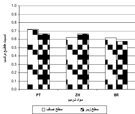
شکل ۲۷- نسبت مقطع مرکب تیرهای خمشی در شرایط عمل آوری ترکیبی
