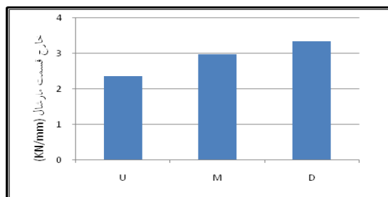
شکل ۴- مقدار خارج قسمت مارشال برای مخلوط‌های با دانه‌بندی‌های مختلف
