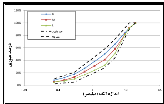
شکل ۱- نمایش دانه‌بندی به روش مرسوم
