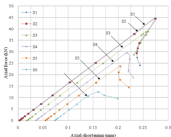
شکل ۲- نمودار جابجایی قائم - نیروی محوری نمونه‌های S1 تا S6
