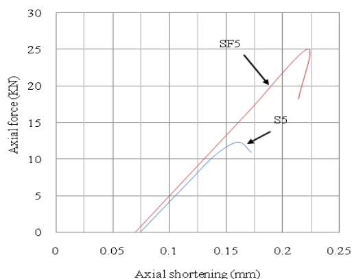
شکل ۶- نمودار مقایسه‌ای جابجایی قائم- نیروی محوری برای نمونه‌های S5 و SF5
