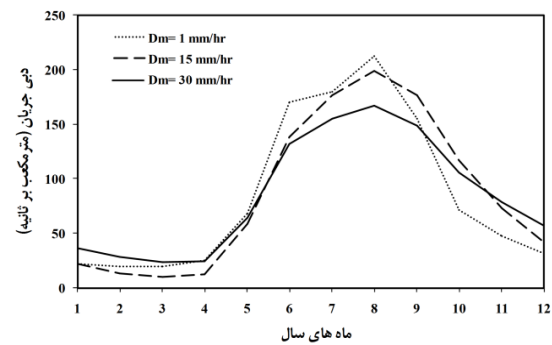
شکل ۲۴- اثر تغییر پارامتر D_m بر هیدروگراف جریان سالانه
