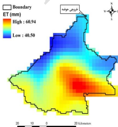
شکل ۹- توزیع مکانی تبخیر و تعرق در ماه تیر
