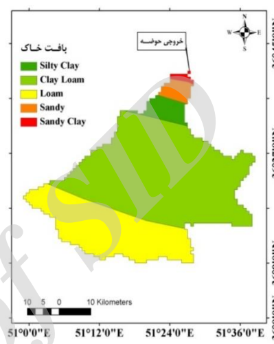
شکل ۴- نقشه بافت خاک حوضه آبریز رودخانه چالوس
