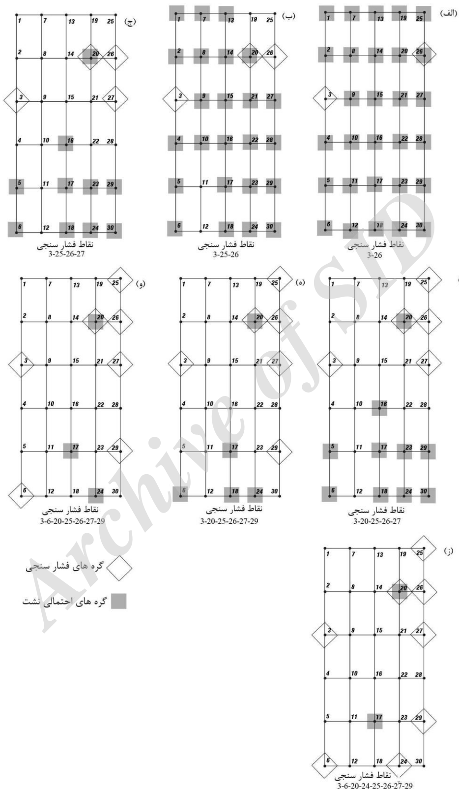
شکل ۴- گره های احتمالی دارای نشت به ازای فشارسنجی های مختلف
