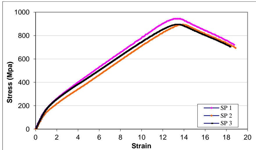
شکل ۲- نمودار تنش بر حسب کرنش میله‌های آزمایش شده در تست کشش
