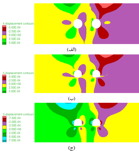
شکل ۱۸- جابجایی افقی ایجاد شده در انتهای حفاری: الف) تونل با مقطع دایره‌ای شکل، ب) تونل با مقطع دوقوسی، ج) تونل با مقطع نعل اسبی شکل
