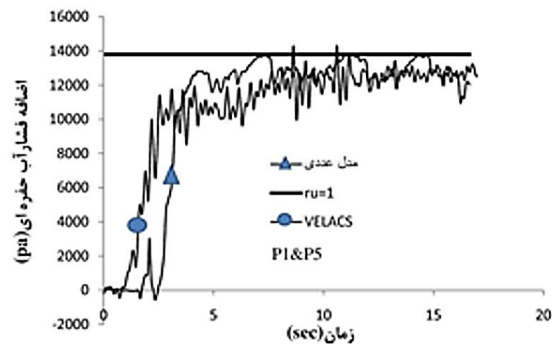
شکل ۴- مقایسه مقادیر اضافه فشار آب حفره‌ای در عمق 1/5m
