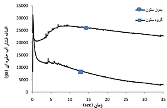
شکل ۱۶- تغییرات اضافه فشار آب حفره ای در برابر زمان
