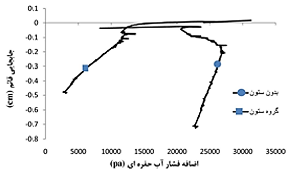
شکل ۱۷- تغییرات جابه جایی قائم در برابر اضافه فشار حفره ای
