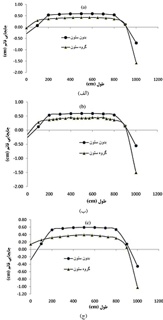
شکل ۱۳- پروفیل طولی خاک در سطح زمین: الف) وسط مدل، ب) ۱ متری از وسط مدل، ج) ۲ متری از وسط مدل
