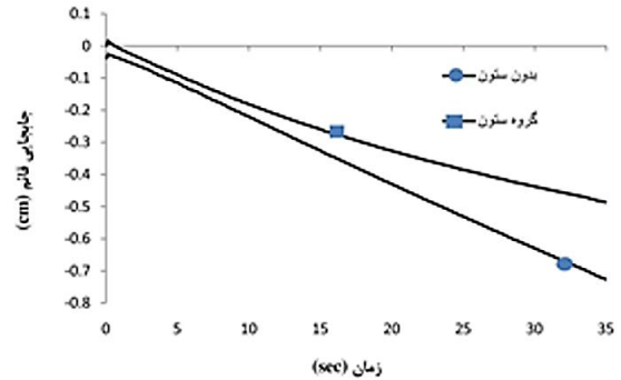
شکل ۱۵- تغییرات جابه جایی قائم در برابر زمان
