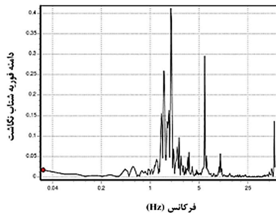
شکل ۳- طیف فوريه شتاب نگاشت قبل از فیلترسازی
