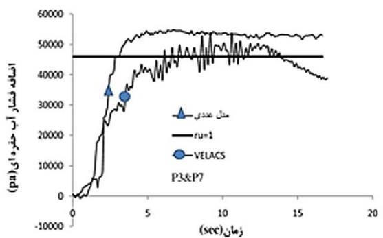
شکل ۶- مقایسه مقادیر اضافه فشار آب حفره‌ای در عمق 5m
