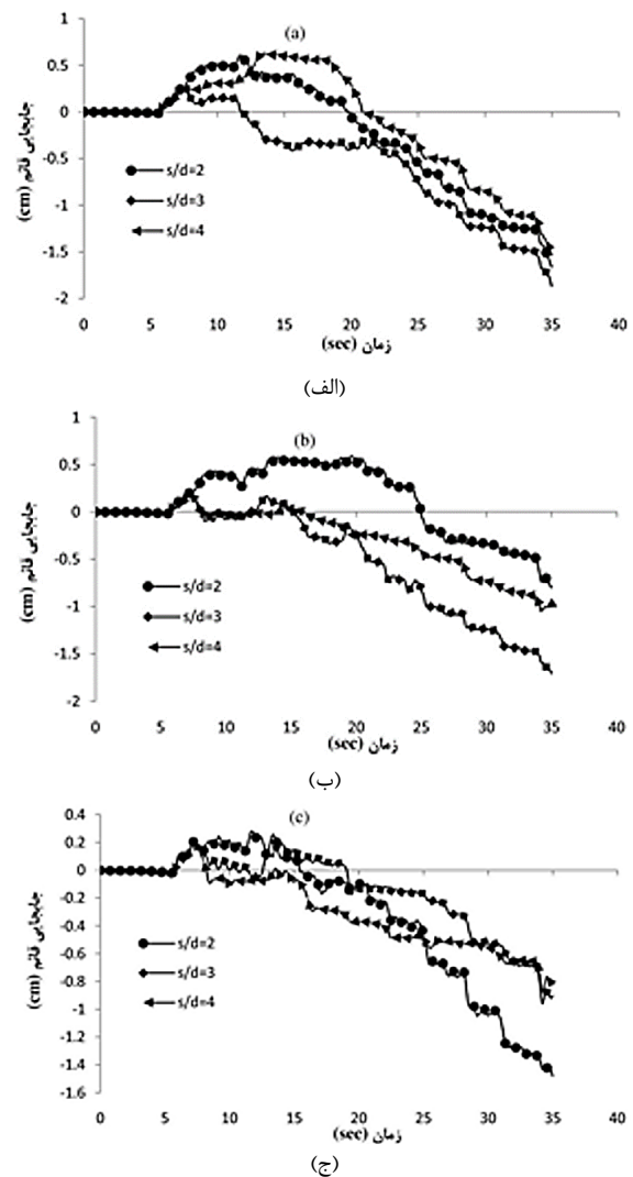
شکل ۱۲- تغییرات جابه جایی قائم (نشست) در سطح زمین برای گروه ستون‌های ۲، ۳ و ۴: الف) قطر ۰/۶ متر، ب) قطر ۱ متر، ج) قطر ۱/۲ متر
