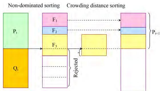
شکل ۱- نحوه مرتب کردن جمعیت در الگوریتم NSGA-II که در آن P_t جمعیت اولیه و Q_t جمعیت ناشی از تقاطع و جهش است و F_i نشان‌دهنده جبهه‌ها است [۶].
