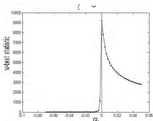
شکل ۶- نمودار مقادیر آماره w-test چند متغیره به ازای مقادیر مختلف \alpha برای نویز گوسی
