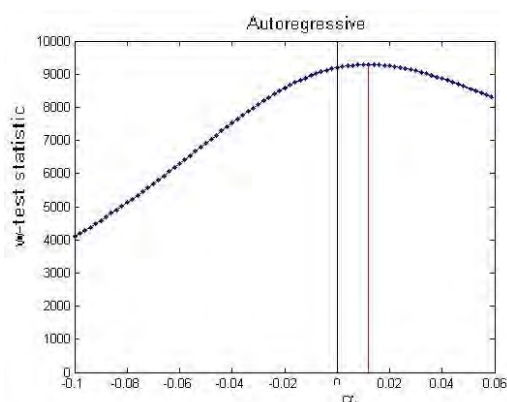
شکل ۴- نمودار مقادیر آماره w-test چند متغیره به ازای مقادیر مختلف \alpha برای نویز اتو-رگسیو
