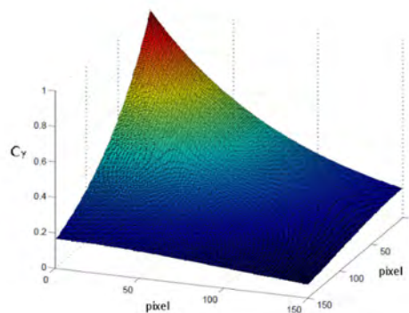
شکل ۹- نمودار دو بعدی نوین اتو-رگرسیون به ازای \alpha برابر ۰٫۰۱۲۰
