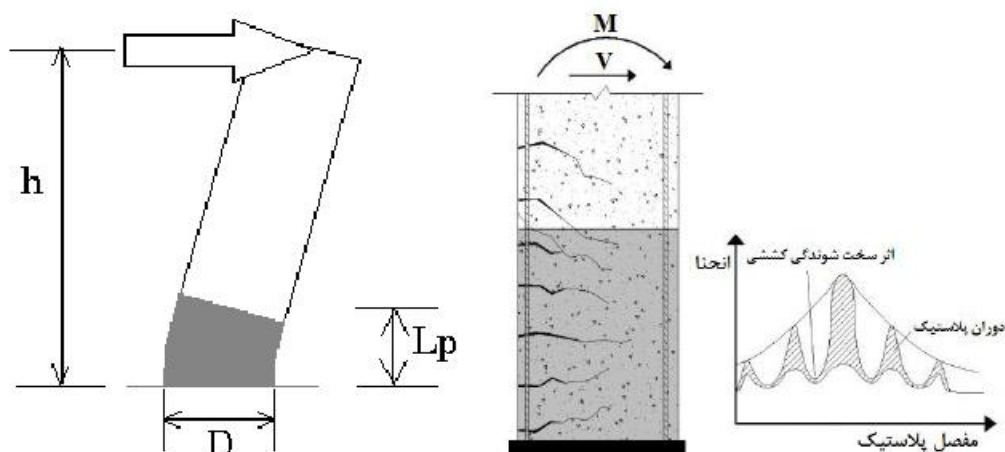
شکل ۱۲. ناحیه مفصل پلاستیک در پایه پل‌های بتن آرمه
