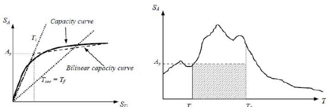
شکل ۵. توصیف نمایشی معیار اندازه گیری شدت طیفی ( I_a )
