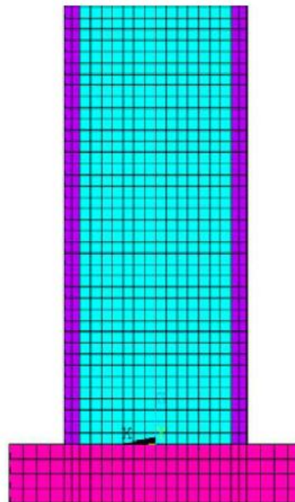
شکل ۹. مدل اجزای محدود نمونه‌های مورد بررسی
