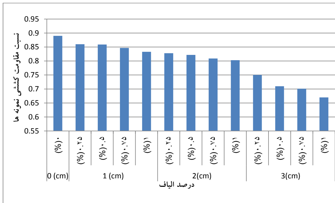
شکل ۷. نسبت مقاومت کششی نمونه‌ها
