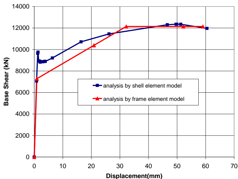
شکل ۱۰. مقایسه رفتار غیرخطی مدل CWPI، به وسیله مدل‌سازی با المان shell و frame در بستر صلب
