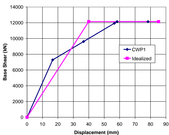
د- منحنی ظرفیت سازه پایه مدل CWP1
