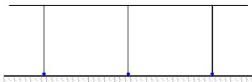
شکل ۵. مدل سازی اثر بستر به وسیله فنرهای الاستیک با سختی مناسب و اختصاص مفاصل برشی به پایه ها
