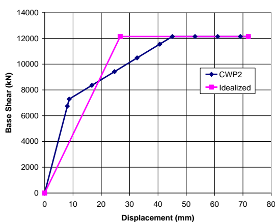
ج- منحنی ظرفیت سازه پایه مدل CWP2
