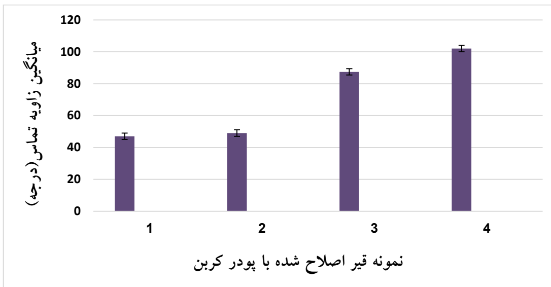
شکل ۵. نتایج آزمایش زاویه تماس برای قیر شاهد و قیرهای اصلاح شده با پودر کربن
