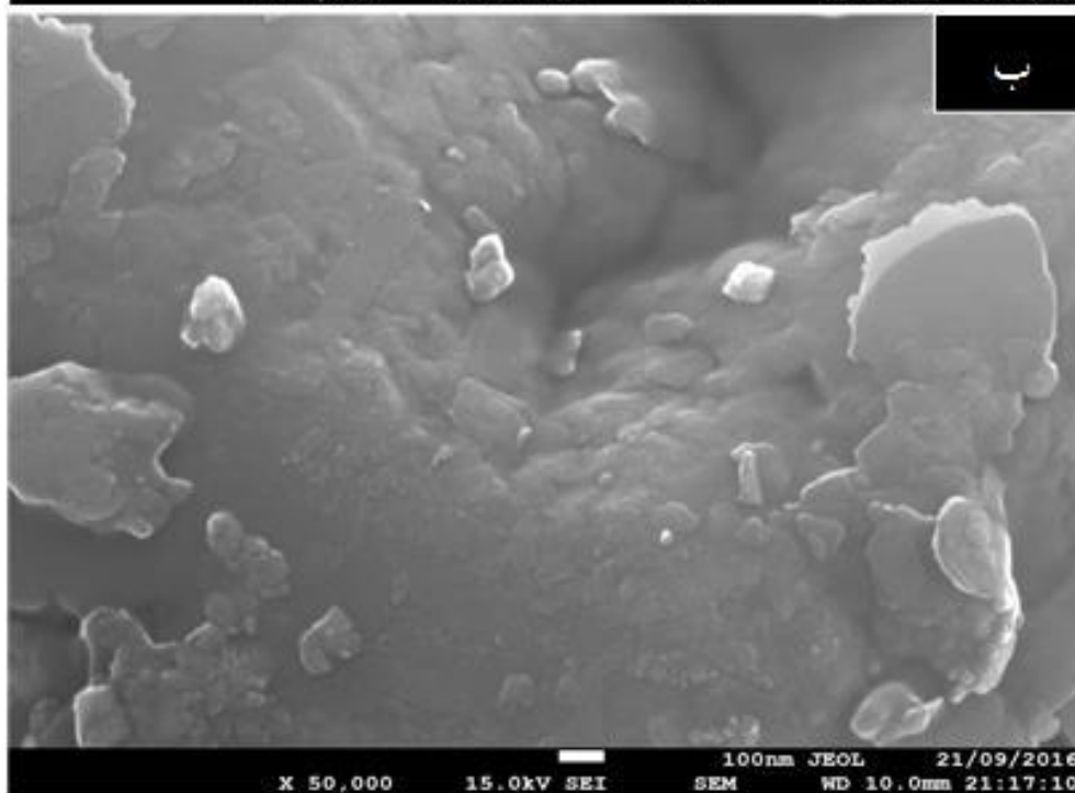
شکل ۱. تصویر SEM: الف) پودر کربن آمورف و ب) پودر سنگ عبوری الک ۲۰۰ (فیلر)
