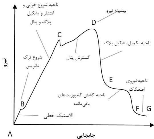
شکل ۹ مراحل مختلف مکانیزم شکست در منحنی نیرو-جابجایی
