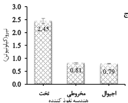
شکل ۱۰ تغییرات نیروی تماسی حداکثر
