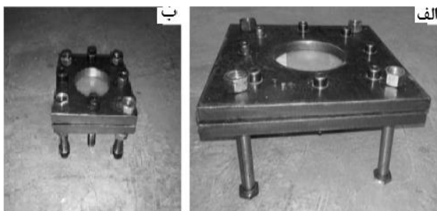
شکل ۳ فیکسچر آزمایش برش پنج نمونه‌های کامپوزیت الف) I=۵ (ب) I=۲/۵
