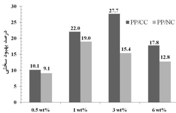
شکل ۲۲ اثر پرکننده بر روی سختی کامپوزیت‌های پلی‌پروپیلن
