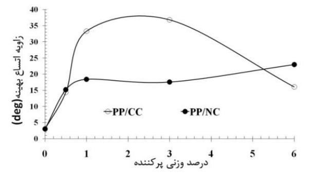
شکل ۳۱ زاویه اتساع محاسبه شده بر اساس بهینه یابی
