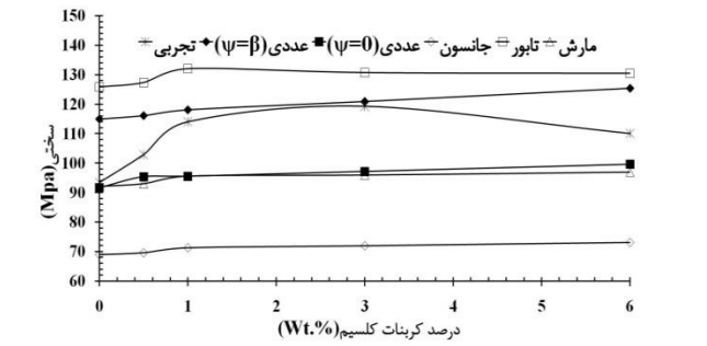
شکل ۳۳ مقایسه سختی کامپوزیت پلی پروپیلن/کربنات کلسیم حاصل از مدل‌های ماکرومکانیکی با نتایج تجربی و عددی
