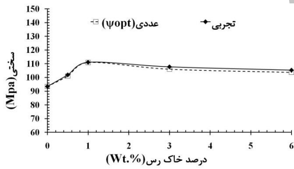
شکل ۳۰ مقایسه سختی کامپوزیت پلی پروپیلن/خاک رس حاصل از روش تجربی و روش عددی (با زاویه اتساع بهینه)
