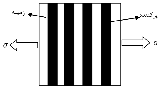
شکل ۱۷ مدل میکرومکانیکی بر اساس معکوس قانون مخلوط‌ها
