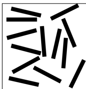
شکل ۱۹ مدل میکرومکانیکی بر اساس مدل هافین-تسای تصادفی
