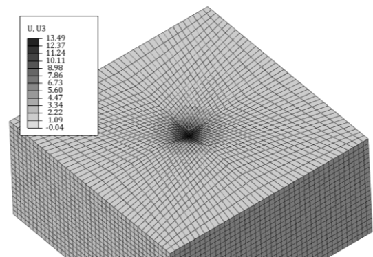
شکل ۱۲ تغییر شکل نمونه پلیمری در آزمون ویکرز
