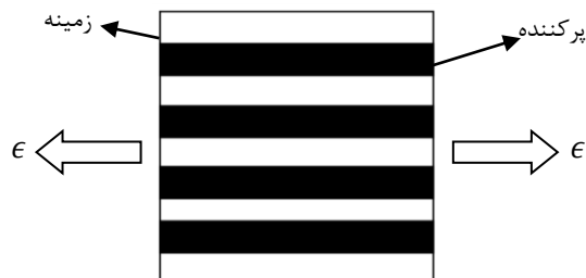
شکل ۱۵ مدل میکرومکانیکی بر اساس قانون مخلوطها
