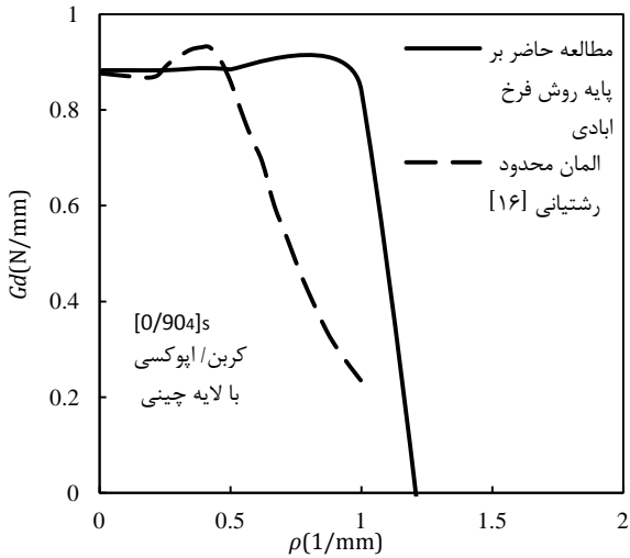
شکل ۲۲ مقایسه نرخ رهایی انرژی کرنشی ناشی از جدایی بین لایه ای به صورت تابعی از چگالی ترک ماتریس در چندلایه حاوی جدایی بین لایه ای و ترک ماتریسی تحت بارگذاری کششی با نسبت \frac{L_d}{L} = 0.1
