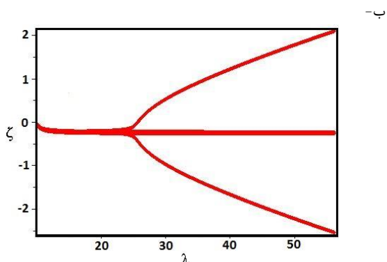
شکل ۷ الف- فرکانس بی بعد فلاتر بر حسب فشار آیرودینامیکی بی بعد ب- دمپینگ بر حسب فشار آیرودینامیکی بی بعد
