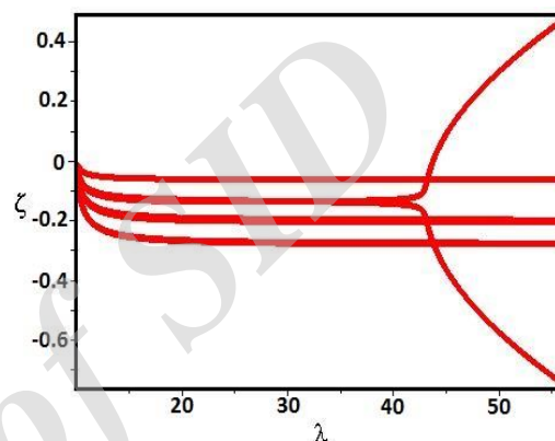
شکل ۹ الف- فرکانس بی بعد فلاتر بر حسب فشار آیرودینامیکی ب- دمینگ بر حسب فشار آیرودینامیکی
