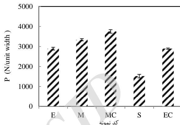
شکل ۹ نمودار میله‌ای استحکام متوسط پوست‌کنی برای پنج نمونه اتصال چسبی نوع E, S, MC و M.
