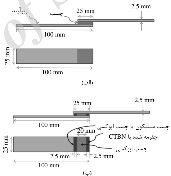
شکل ۱ نمونه آزمون تک لبه‌ای برشی (الف) اتصال تک لبه‌ای ساده و (ب) اتصال تک لبه‌ای با چسب ترکیبی
