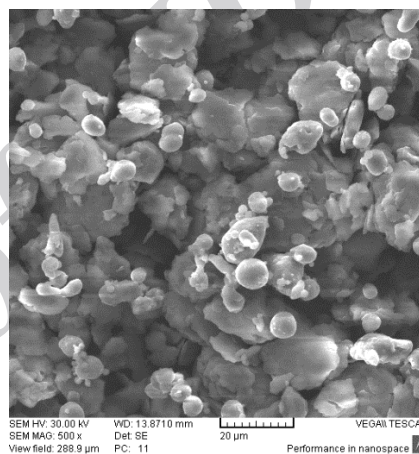
Fig. 3 The pure Al powder after 36 h of ball-milling process شکل 3 ذرات آلومینیوم خالص بعد از 36 ساعت آسیاب مکانیکی
