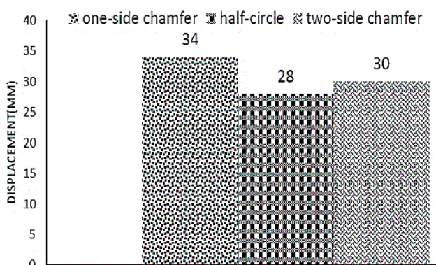
Fig. 33 Destruction value for testing the end shape of the sample شکل 33 مقدار تخریب برای آزمایش شکل انتهای نمونه
