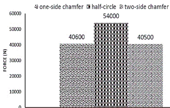
Fig. 32. Force value in first area for testing the end shape of the sample شکل 32 مقدار نیرو در ناحیه 1 برای آزمایش شکل انتهای نمونه
