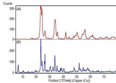
شکل ۴. الگوی پراش اشعه ایکس نمونه‌های لایه نازک آماده شده با استفاده از سل حاوی کمپلکس اسید آگزالیک با حضور لوریک الکل (A) و بدون آن (B).
