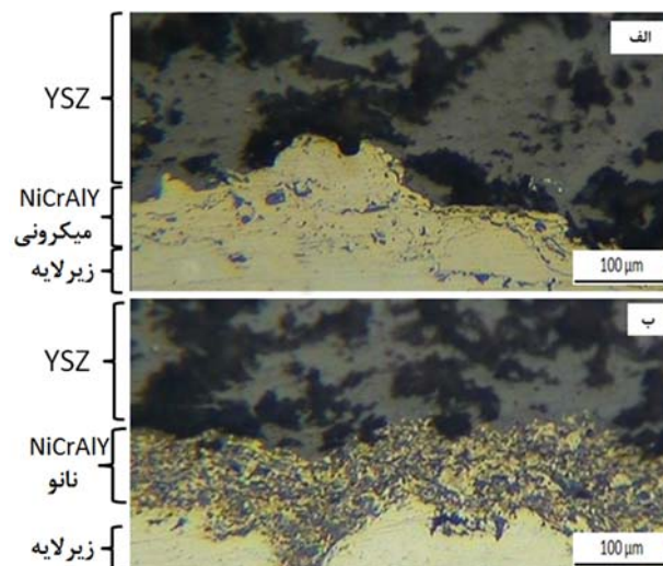
شکل ۲. لایه پیوندی ایجاد شده از: (الف) پودر میکرونی NiCrAlY (ب) پودر نانو NiCrAlY آگلومره شده.
