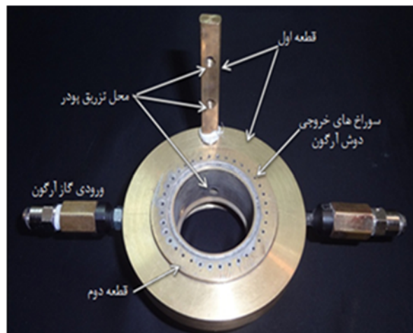
شکل ۱. تصویر قطعات طراحی شده و اجزای آن‌ها.
