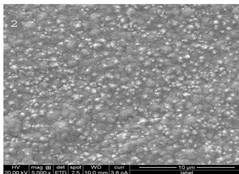
شکل ۱. تصاویر میکروسکوپی از پوشش های (۱) نیکل (۲) Ni-Graphene در حمام واتر [۵].
