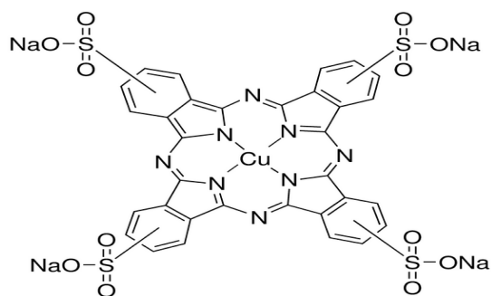
شکل ۱. ساختار فتالوسیانین مس سولفونه شده.
