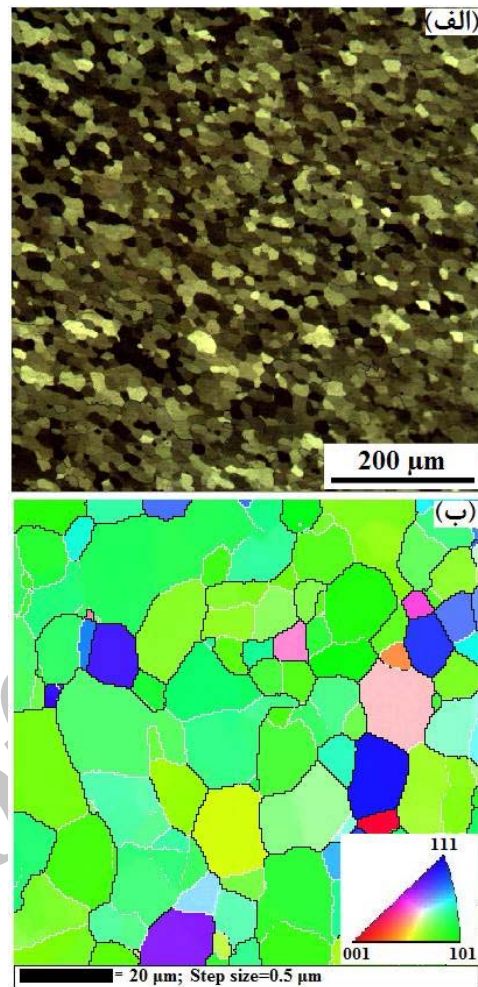
شکل ۳. تصویر (الف) میکروسکوپ نوری و (ب) EBSD از منطقه اغتشاش یافته نمونه فرآوری شده در دمای اتاق و بدون نانوذرات.
