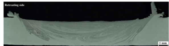
شکل ۴. سطح مقطع نمونه فرآوری شده با سه پاس فرآیند اصطکاکی اغتشاشی در محیط نیتروژن مایع به همراه نانوذرات SiC.
