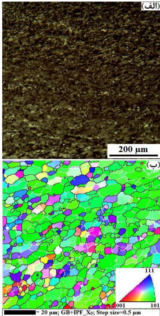
شکل ۵. (الف) تصویر میکروسکوپ نوری و (ب) تصویر EBSD از منطقه اغتشاش یافته نمونه فرآوری شده با سه پاس فرآیند اصطکاکی اغتشاشی در محیط نیتروژن مایع به همراه نانوذرات.
