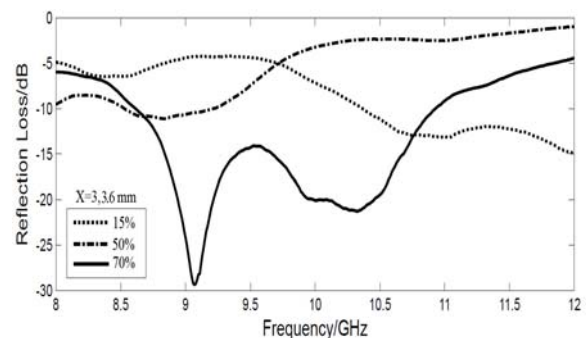
شکل ۴. تاثیر درصد پودر جاذب برای نمونه‌هایی با ضخامت یکسان ۳/۶ میلی‌متر در باند X.
