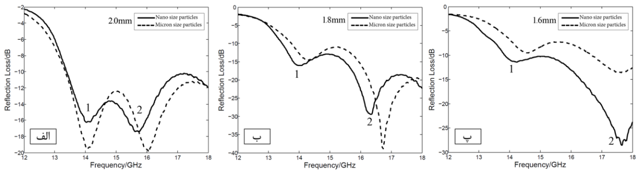
شکل ۷. بررسی تاثیر اندازه ذرات در الگوی جذب در ضخامت‌های ۱/۶، ۱/۸، و ۲/۰ میلی‌متر در بازه فرکانسی ۱۲-۱۸ گیگاهرتز، BaFe_9Mg_{1.5}Ti_{1.5}O_{19} .
