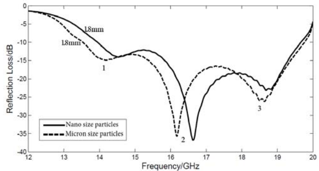
شکل ۹. بررسی تاثیر اندازه ذرات در الگوی جذب نمونه‌ای با ضخامت ۱٫۸ میلی‌متر در بازه فرکانسی ۱۲-۲۰ گیگاهرتز.
