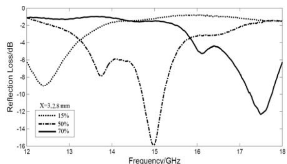
شکل ۵. تاثیر درصد پودر جاذب برای نمونه‌هایی با ضخامت یکسان ۲/۸ میلی‌متر در باند Ku.
