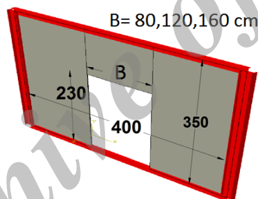
شکل ۷: قاب مورد تحلیل بدون FRP
