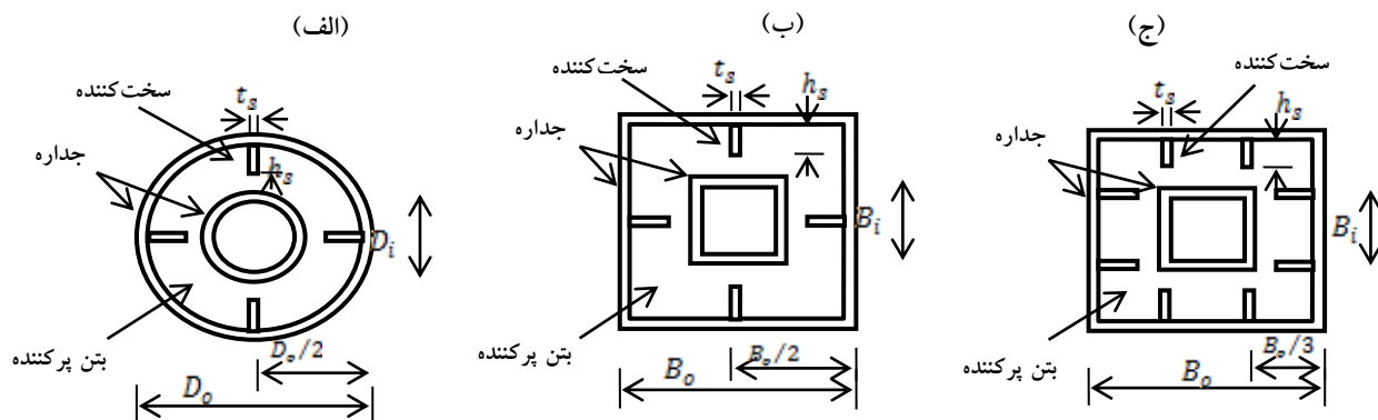
شکل ۶: جزئیات ستون‌های CFDST با افزودن سخت‌کننده: الف) مقطع دایره با سخت‌کننده، ب) مقطع مربع با یک سخت‌کننده در هر وجه،
