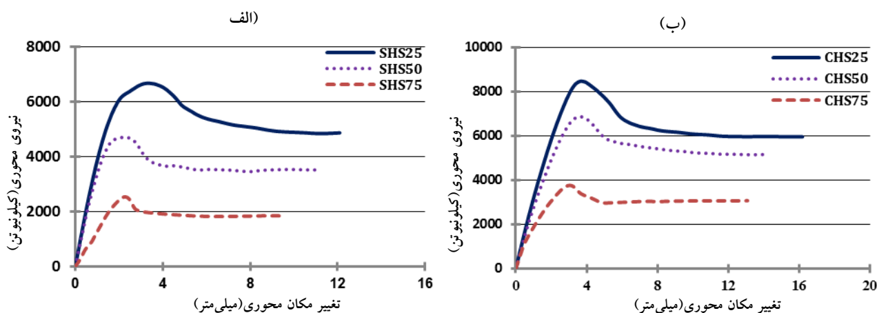
شکل ۸: نمودار نیروی محوری- تغییر مکان محوری ستون‌های CFDST با نسبت‌های توخالی ۰/۰۵۰/۲۵ و ۰/۷۵: الف) مقطع مربع، ب) مقطع دایره
