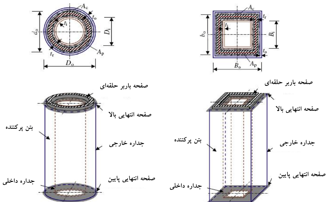
شکل ۲: مدل تحلیلی عناصر محدود با CFDST با مقطع مربع و دایره [۷]
