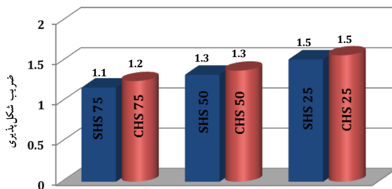
شکل ۱۰: مقایسه ضریب شکل پذیری مقاطع مربع و دایره شکل ستون‌های CFDST با نسبت‌های توخالی ۰/۲۵، ۰/۵۰ و ۰/۷۵
