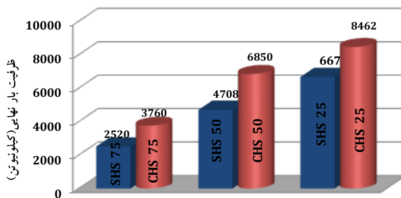
شکل ۹: مقایسه ظرفیت باربری نهایی مقاطع مربع و دایره شکل ستون‌های CFDST با نسبت‌های توخالی ۰/۰۵۰/۲۵ و ۰/۷۵
