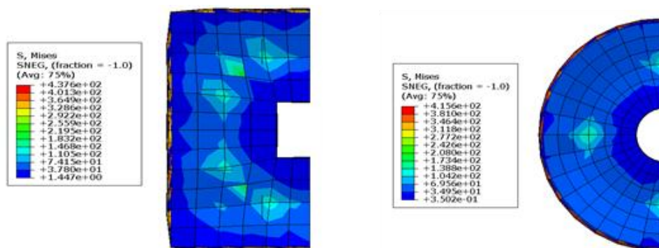
شکل ۱۱: تغییر شکل یافته نمونه‌های CFDST مربع و دایره شکل با افزودن سخت‌کننده
