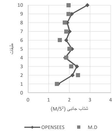
شکل ۹: مقایسه پاسخ شتاب جانبی حاصل از تحلیل تاریخچه زمانی در نرم افزار با شتاب حاصل از رابطه ارائه شده - قاب ۱۰ طبقه - زلزله کرن کانتی
