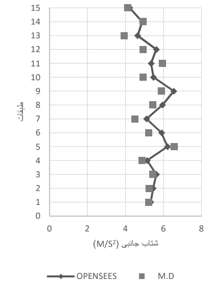
شکل ۱۳: مقایسه پاسخ شتاب جانبی حاصل از تحلیل تاریخچه زمانی در نرم افزار با شتاب حاصل از رابطه ارائه شده - قاب ۱۵ طبقه - زلزله کرن کانتی
