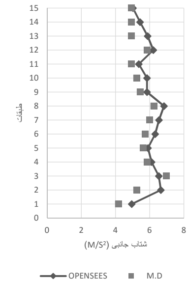
شکل ۱۲: مقایسه پاسخ شتاب جانبی حاصل از تحلیل تاریخچه زمانی در نرم افزار با شتاب حاصل از رابطه ارائه شده - قاب ۱۵ طبقه - زلزله لوماپریتا
