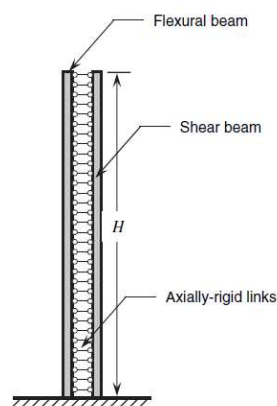
شکل ۴: اتصالات در مدل ساده تیر طره [۱۱].
