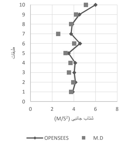
شکل ۱۰: مقایسه پاسخ شتاب جانبی حاصل از تحلیل تاریخچه زمانی در نرم افزار با شتاب حاصل از رابطه ارائه شده - قاب ۱۰ طبقه - زلزله ایمپریال ولی
