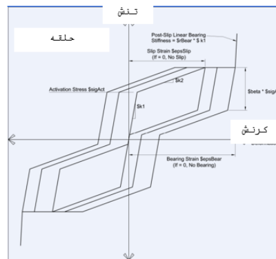
شکل ۷: پارامترهای ماده یک‌جهتی خود مرکز [۱۳].
