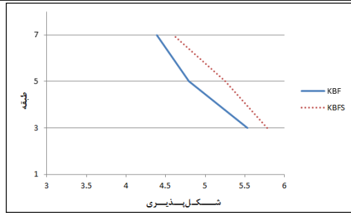
شکل ۱۱: مقایسه مقدار ظرفیت شکل‌پذیری در قاب‌ها.
