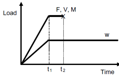
شکل ۶: تاریخچه زمانی بارگذاری [۲۲].
