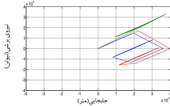
شکل ۱۵: نمودار نیرو-جابجایی جداساز ۱ (قرمز) جداساز ۲ (سبز) جداساز ۳ (آبی)
