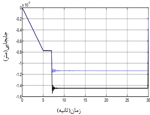
ب: جابجایی قائم سرستون در گره ۶
