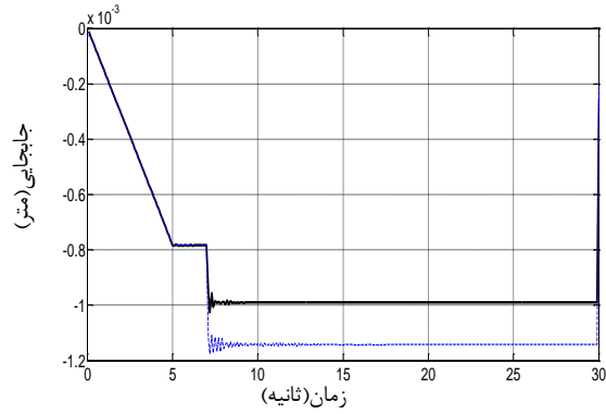
الف: جابجایی قائم سرستون در گره ۴
