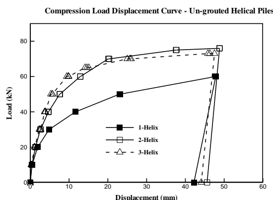
شکل ۱۱: نتایج آزمایش بارگذاری شمع های بدون تزریق در سایت.
