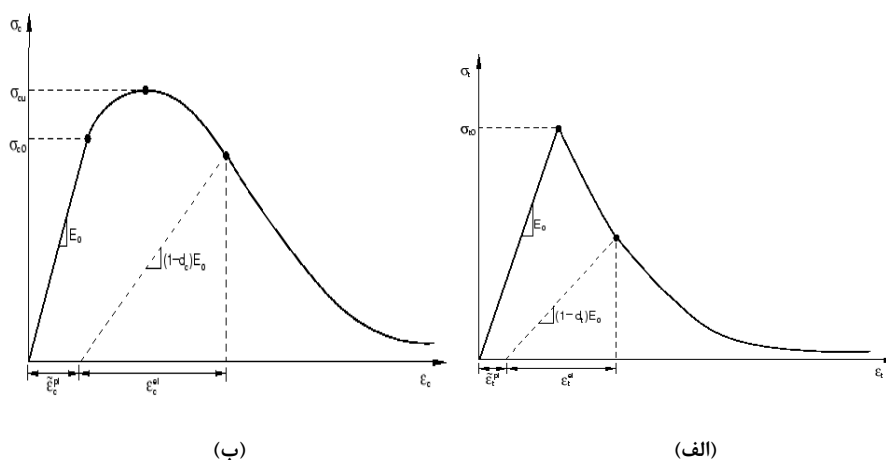
شکل ۲: رفتار بتن در برابر بارگذاری تک محوره [۱۴].
