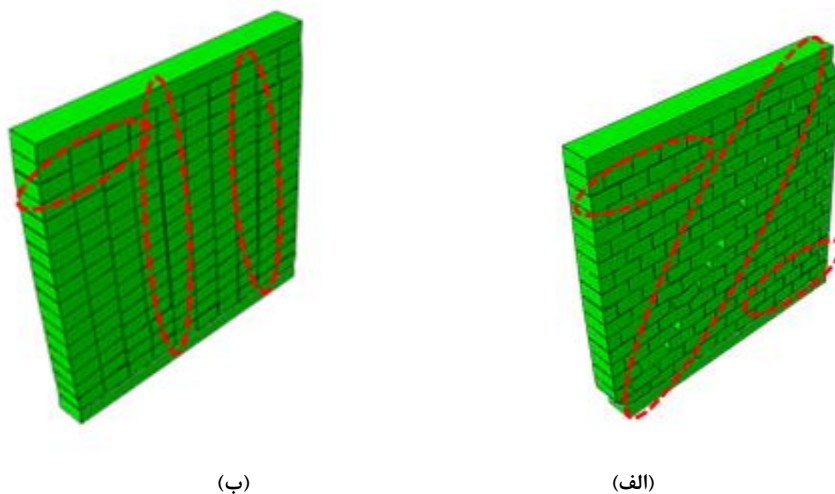
شکل ۱۲: مد خرابی دیوار بنایی، (الف) پیوند انگلیسی، (ب) پیوند انباشته.
