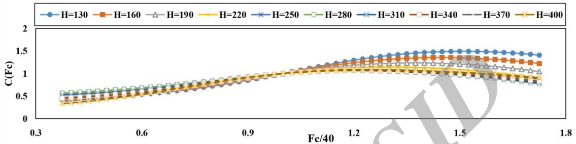
شکل ۱۰: ضریب اصلاحی C(F_c) برای مقادیر مختلف H
