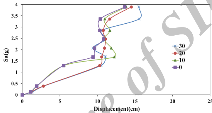
سه دهانه
