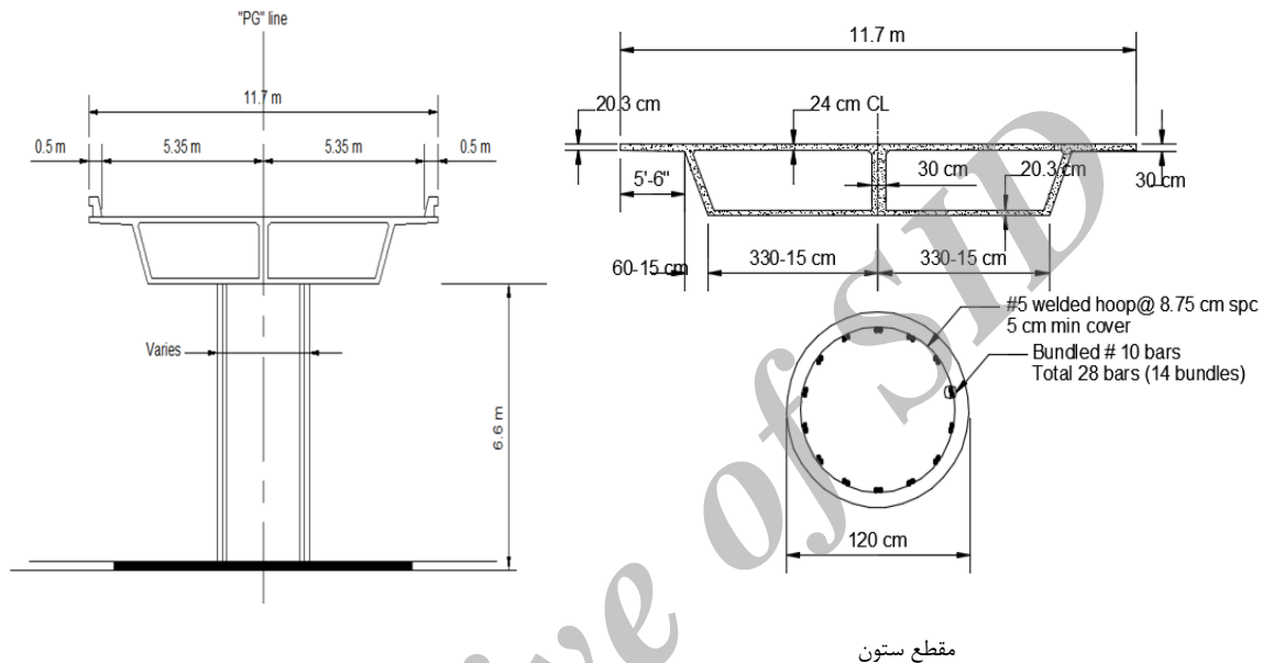
مقطع ستون
