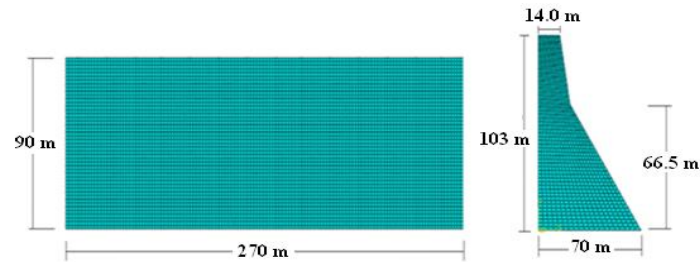
شکل ۷: مدل المان محدود سد - مخزن، سد بتنی وزنی کوینا مورد استفاده در صحت سنجی
