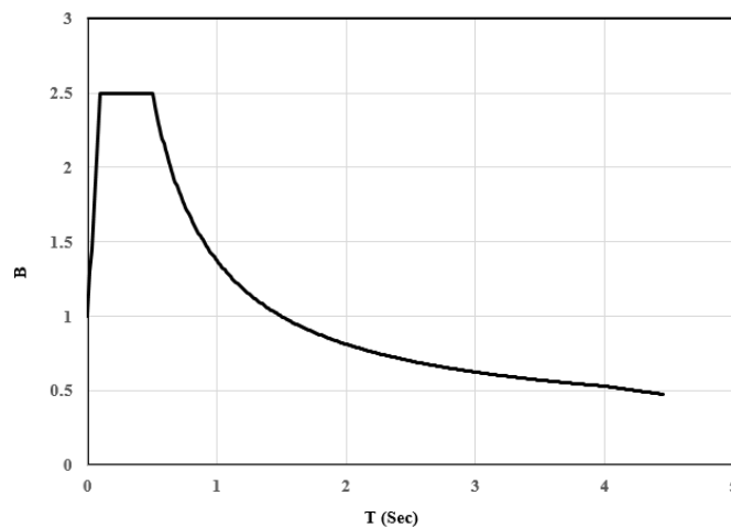
شکل ۵: منحنی ضریب بازتاب مربوط به ساختگاه با خاک نوع ۲
