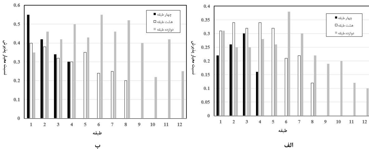
شکل ۶: مقدار حداکثر نسبت معیار پذیرش بحرانی ستون ها در ساختمان های ۴، ۸ و ۱۲ طبقه، الف- شکل پذیري ویژه ب- شکل پذیري متوسط
