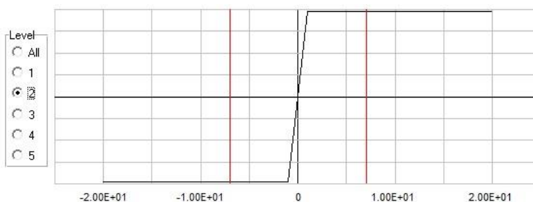
شکل ۸: نمونه ای از مفاصل خمیری تعریف شده در نرم افزار Perform 3D برای تیرها
