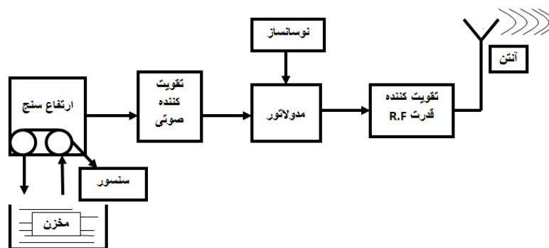
شکل ۳: بلوک دیاگرام ایستگاه‌های ۱ و ۲
