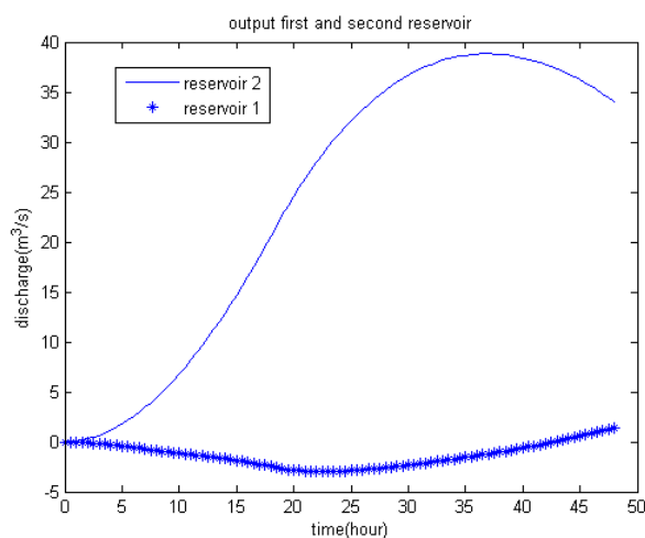
شکل ۱۲: دبی خروج از مخازن ۲ و ۱
