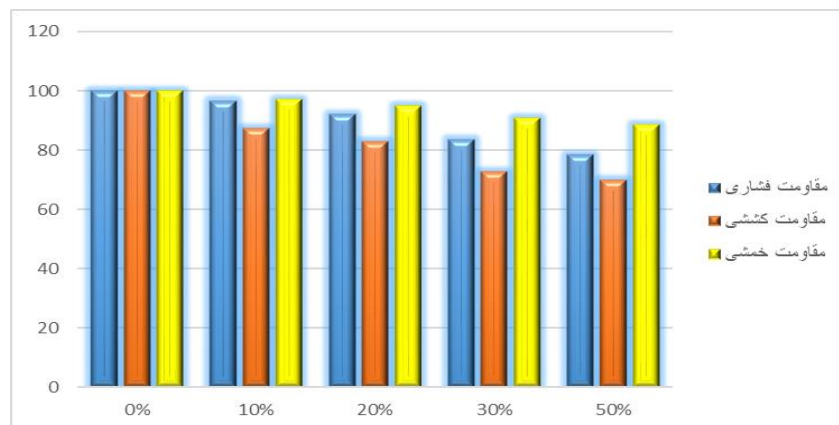
شکل ۱۰ - مقایسه درصد مقاومت فشاری، کششی و خمشی در حالت ۲۸ روزه
