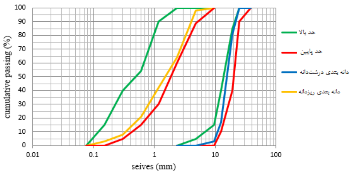
شکل ۱ نمودار دانه‌بندی
