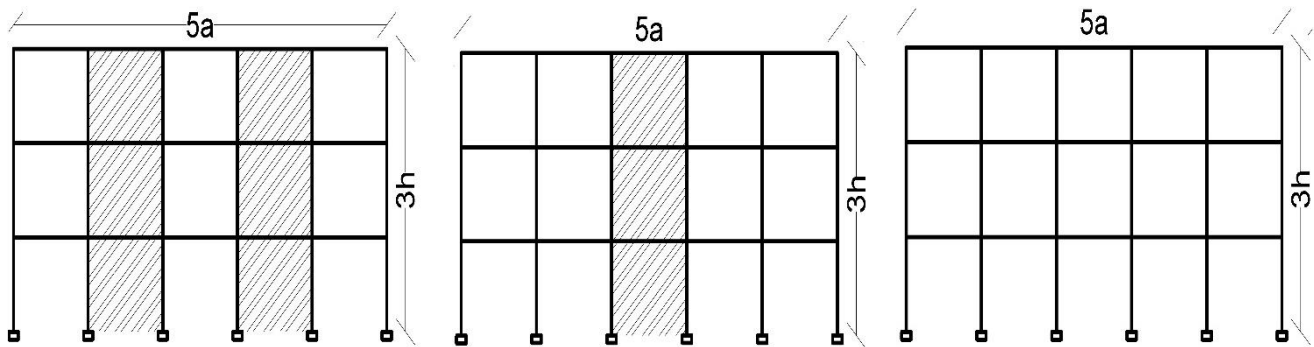
الف) قاب خمشی فولادی ویژه ب) قاب فولادی با ۱ دهانه دیوار برشی فولادی ج) قاب فولادی با ۲ دهانه دیوار برشی فولادی
