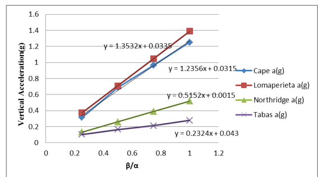
شکل ۴: حداکثر شتاب قائم پوشش تونل در بارگذاری ۱ تا ۴
