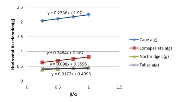
شکل ۵: حداکثر شتاب افقی پوشش تونل در بارگذاری ۱ تا ۴
