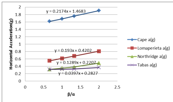
شکل ۶: حداکثر شتاب افقی پوشش تونل در بارگذاری ۵ تا ۸
