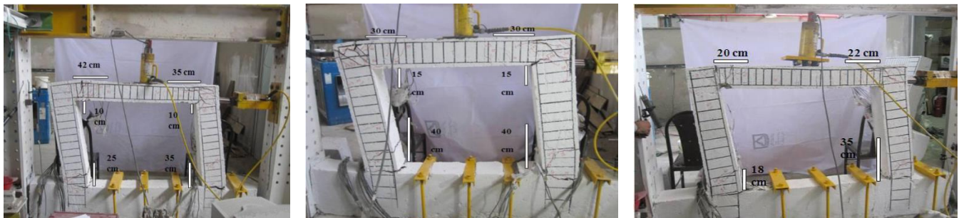
شکل ۱۳: نحوه شکست قاب‌ها تحت آزمایش بارگذاری جانبی افزایشی [2]، الف: قاب RC ب: قاب RCH ج: قاب RH
