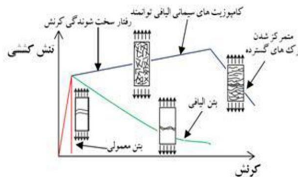
شکل ۱: مقایسه رفتار کششی بتن معمولی، FRC و HPFRCC
