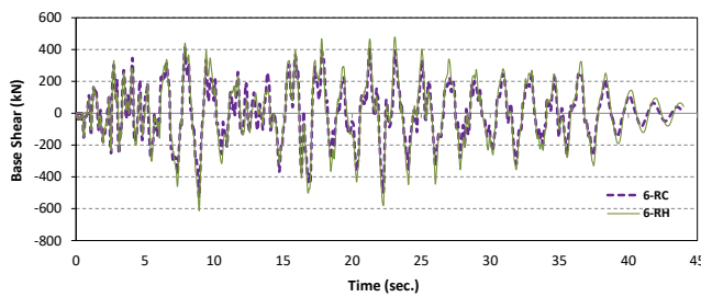
ب) قاب ۶ طبقه (زلزله لندرز)
