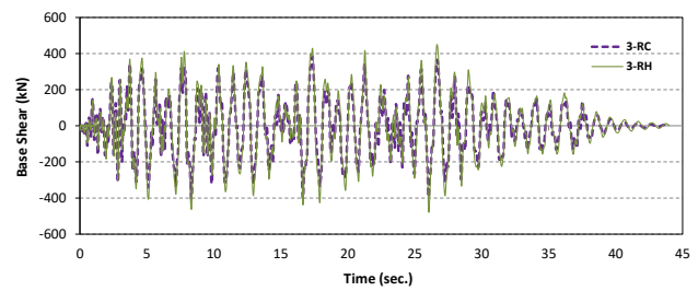
الف) قاب ۳ طبقه (زلزله لندرز)
