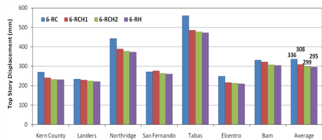
ج) قاب ۶ طبقه، زلزله سطح خطر یک
