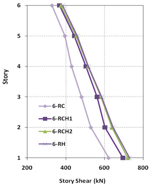
د) قاب‌های ۶ طبقه زلزله سطح خطر دو
