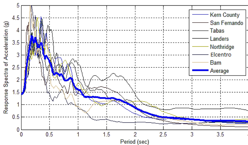
شکل ۱۷: متوسط‌گیری طیف پاسخ شتاب شتاب‌نگاشت‌ها
