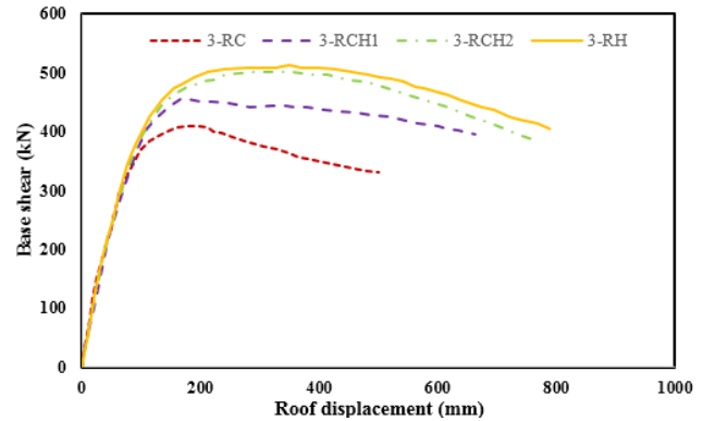
الف) قاب ۳ طبقه
