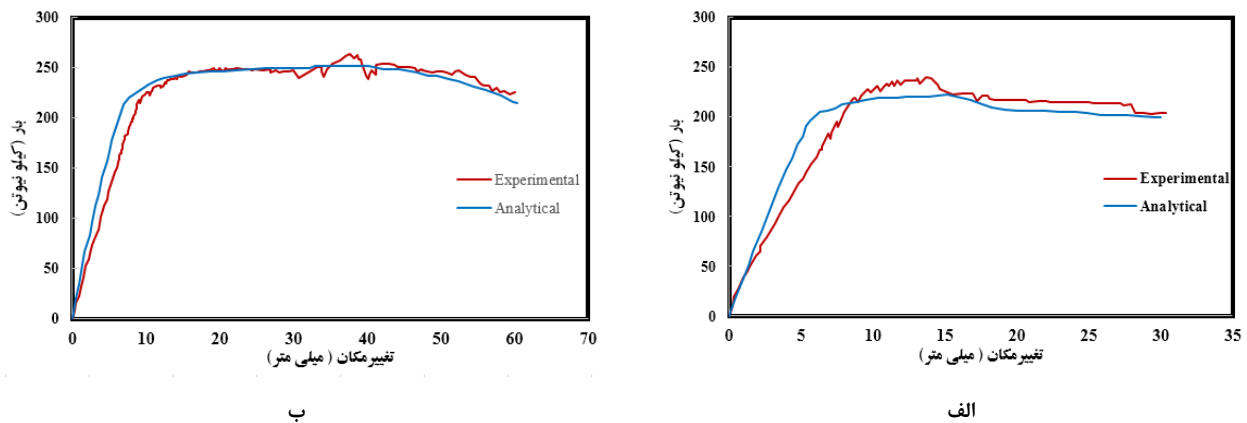
شکل ۱۰: منحنی نیرو- تغییرمکان وسط دهانه ناشی از نتایج آزمایشگاهی [2] و تحلیلی، الف: تیر RC ب: تیر RH
