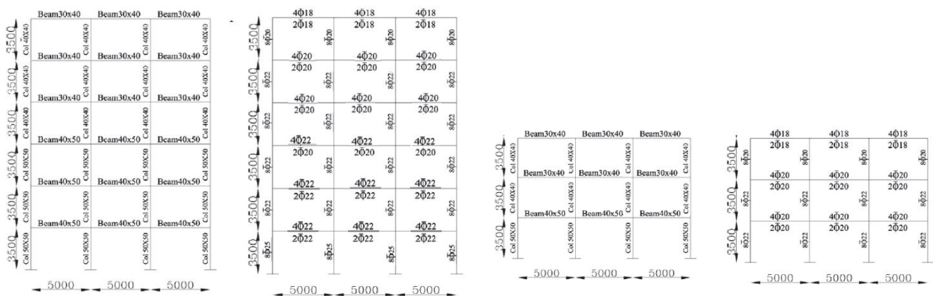
ب) قاب ۳ طبقه ج) قاب ۶ طبقه شکل ۱۴: جزئیات آرمانورگذاری و ابعاد قاب‌های مورد بررسی ۳ و ۶ طبقه (ابعاد برحسب میلی‌متر)
