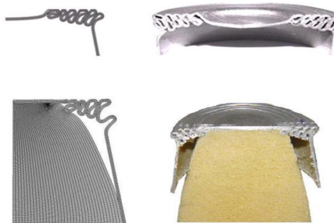
شکل ۴: فروریزش پوسته مخروطی توخالی و تقویت شده با فوم پلی یورتان تحت بارگذاری محوری
