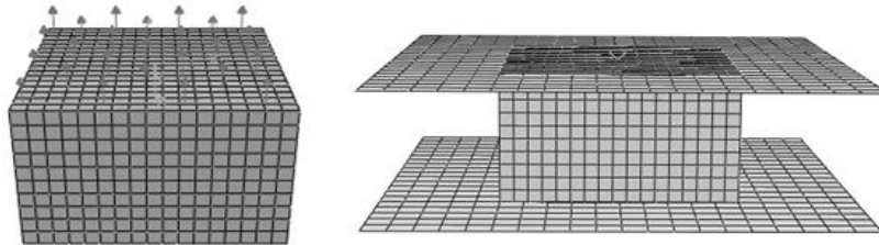
شکل ۱: مدل مورد استفاده برای شبیه‌سازی رفتار مکانیکی الف- فوم پلی‌یورتان و ب- ورق تخت آلومینیوم
