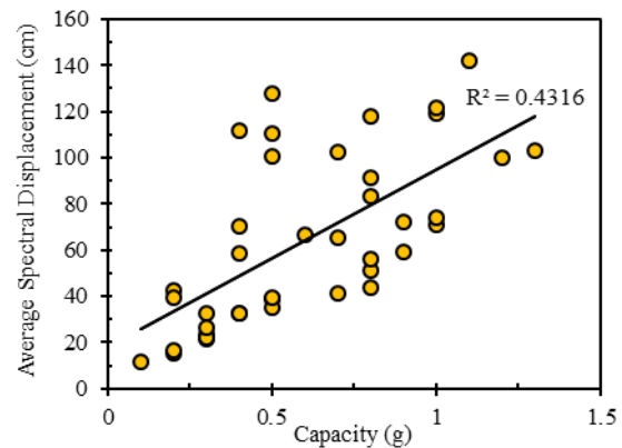
شکل ۱۱: ارتباط بین سنج‌های شدت و حداکثر ظرفیت سازه با بیشترین همبستگی در قاب خمشی ۲۰ طبقه.
