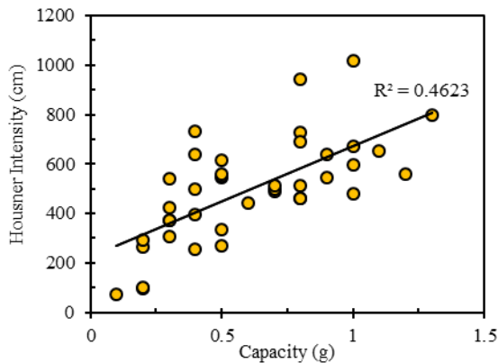
شکل ۱۱: ارتباط بین سنج‌های شدت و حداکثر ظرفیت سازه با بیشترین همبستگی در قاب خمشی ۲۰ طبقه.
