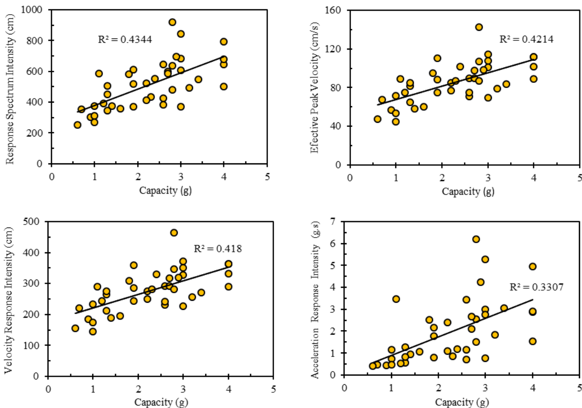
شکل ۸: ارتباط بین سنج‌های شدت و حداکثر ظرفیت سازه با بیشترین همبستگی در قاب خمشی ۴ طبقه.
