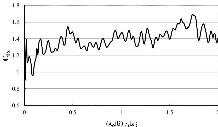
شکل ۵: منحنی تاریخچه زمانی ضریب آئرو دینامیکی C_{Fx}
