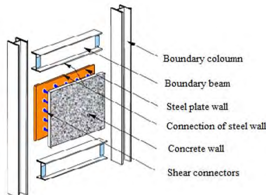
شکل ۱: اجزای اصلی دیوار برشی فولادی مرکب [۱]
