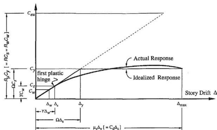
شکل ۱۲: پاسخ عمومی سازه
