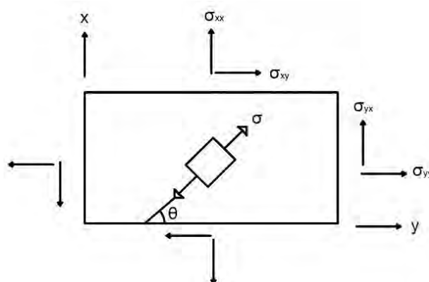
شکل ۱۰: زاویه میدان کششی ورق فولادی [۲]
